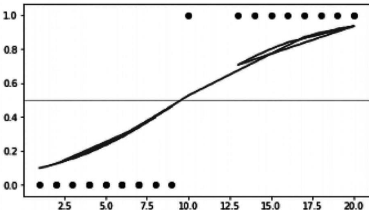
Fig. 9.4 Sigmoid Function
